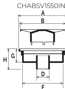
sortie verticale
