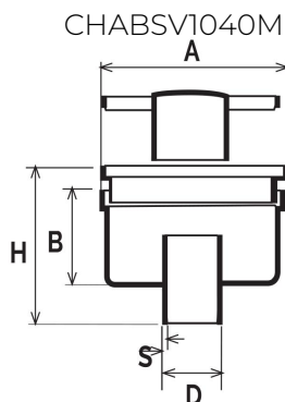
sortie verticale
